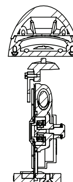
SEZIONE A-A
